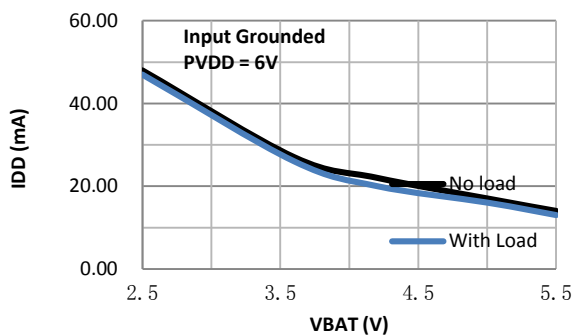
V BAT vs I DD
