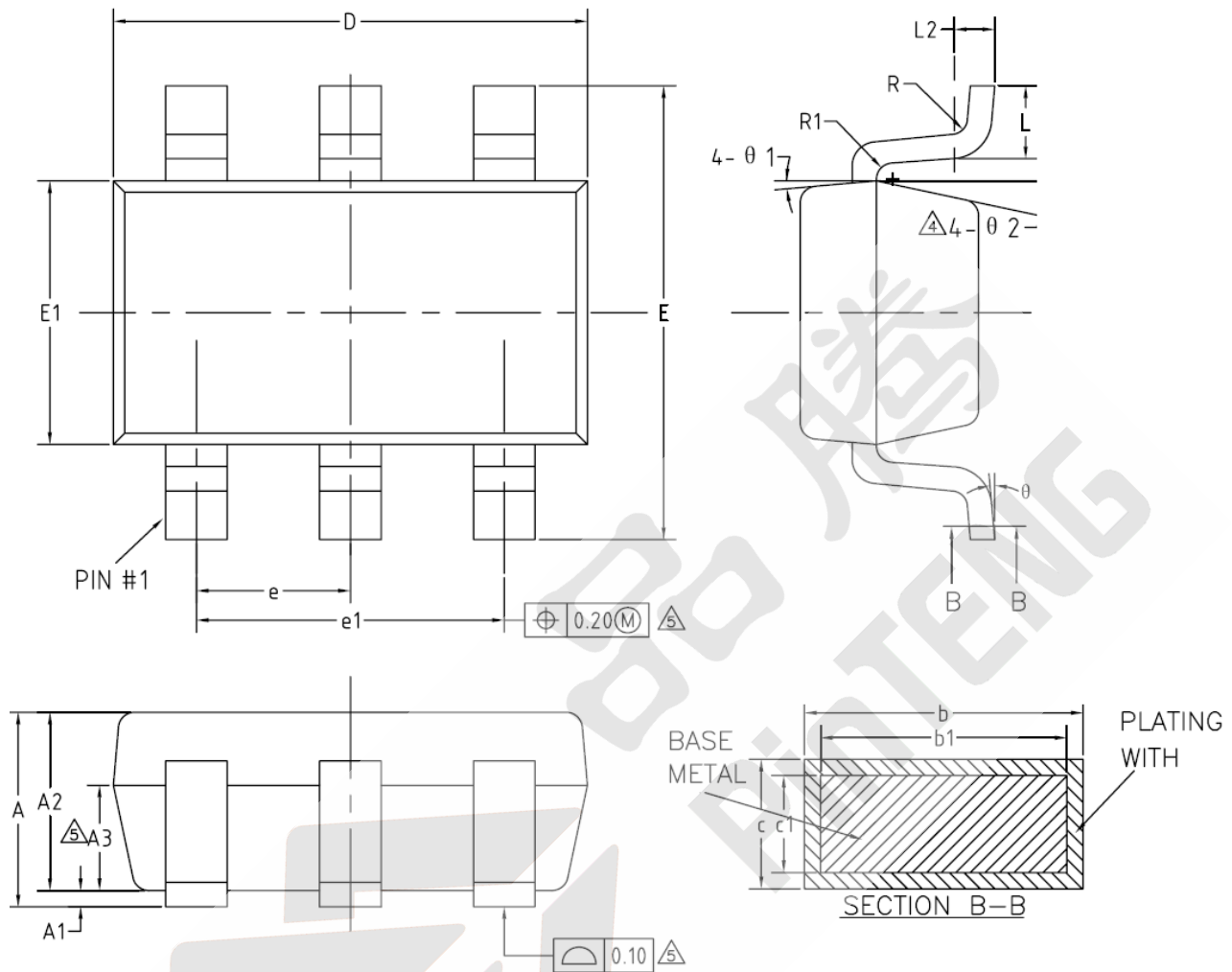
图 7 SOT23-6 封装图
