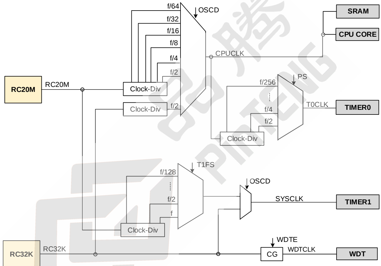
图 4 时钟结构图
