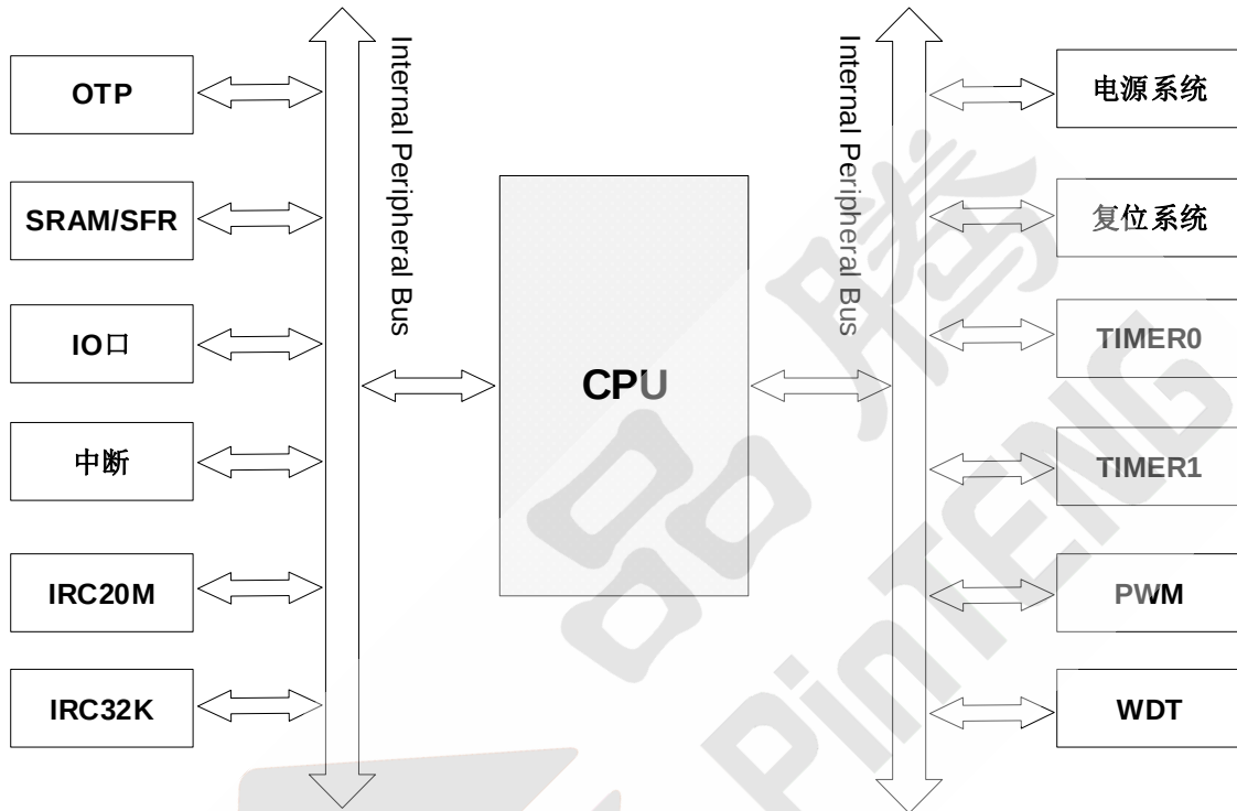
图 2 系统框图
