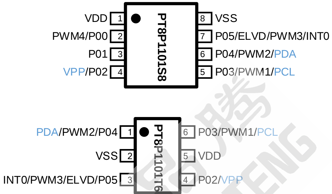
图 1 管脚示意图
